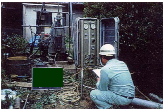
LLT試験状況
